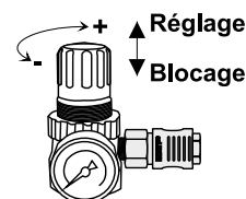
Détendeur
