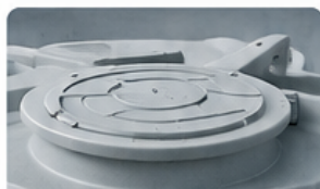
Grand couvercle Ø 600 mm avec ventilation intégrée
