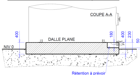
Plan de dalle pour vidange totale
