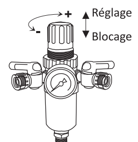
Epurateur-détendeur
