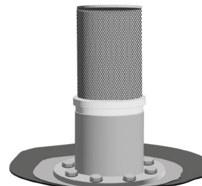
Vidange par le fond Bloc bride INOX boulonné Crépine INOX Manchon PVC-P 110 x 4" (raccordement tuyauterie enterrée à coller)
